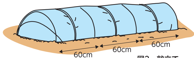
図2 畝立て
